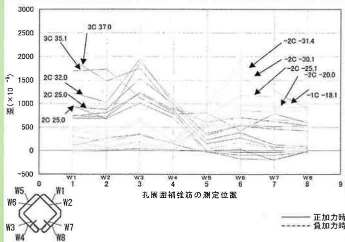
図3 MAX ウェブレンのひずみ (写真1)
