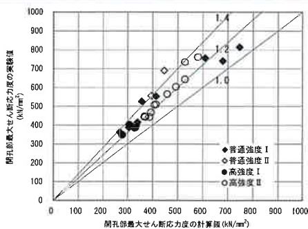
図2 実験値とMAX ウェブレン算定式の値の関係
